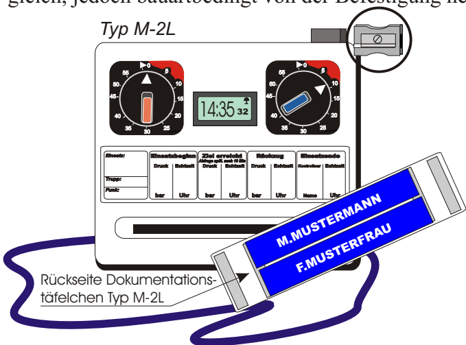
Typ M-2L (Rückseite mit Tabelle und neu jetyt mit Klettstreifen für Ersatztäfelchen)
